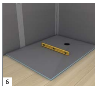
Contrôler le niveau d'écoulement de l'élément wedi Fundo Ligno et l'ajuster éventuellement.
