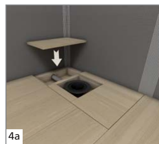
4a Combler les espaces vides avec un aggloméré marine ou un OSB.
