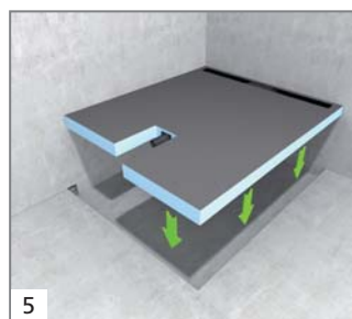
5 Coller l'élément dans la réservation prévue.
