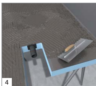
4 Puis poser le receveur par double encollage en utilisant un peigne en denture de 10 mm.
