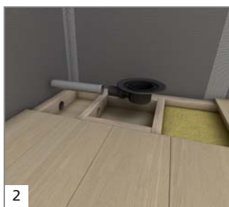
2 Réaliser un chevêtre à l'emplacement du corps du siphon (35 x 35 cm)...
