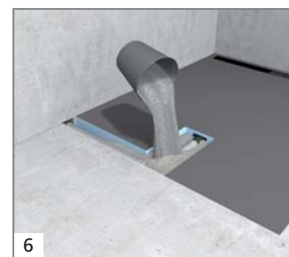
6 ... et raccorder la tuyauterie. Ensuite remplir l'ouverture avec un mortier de scellement.
